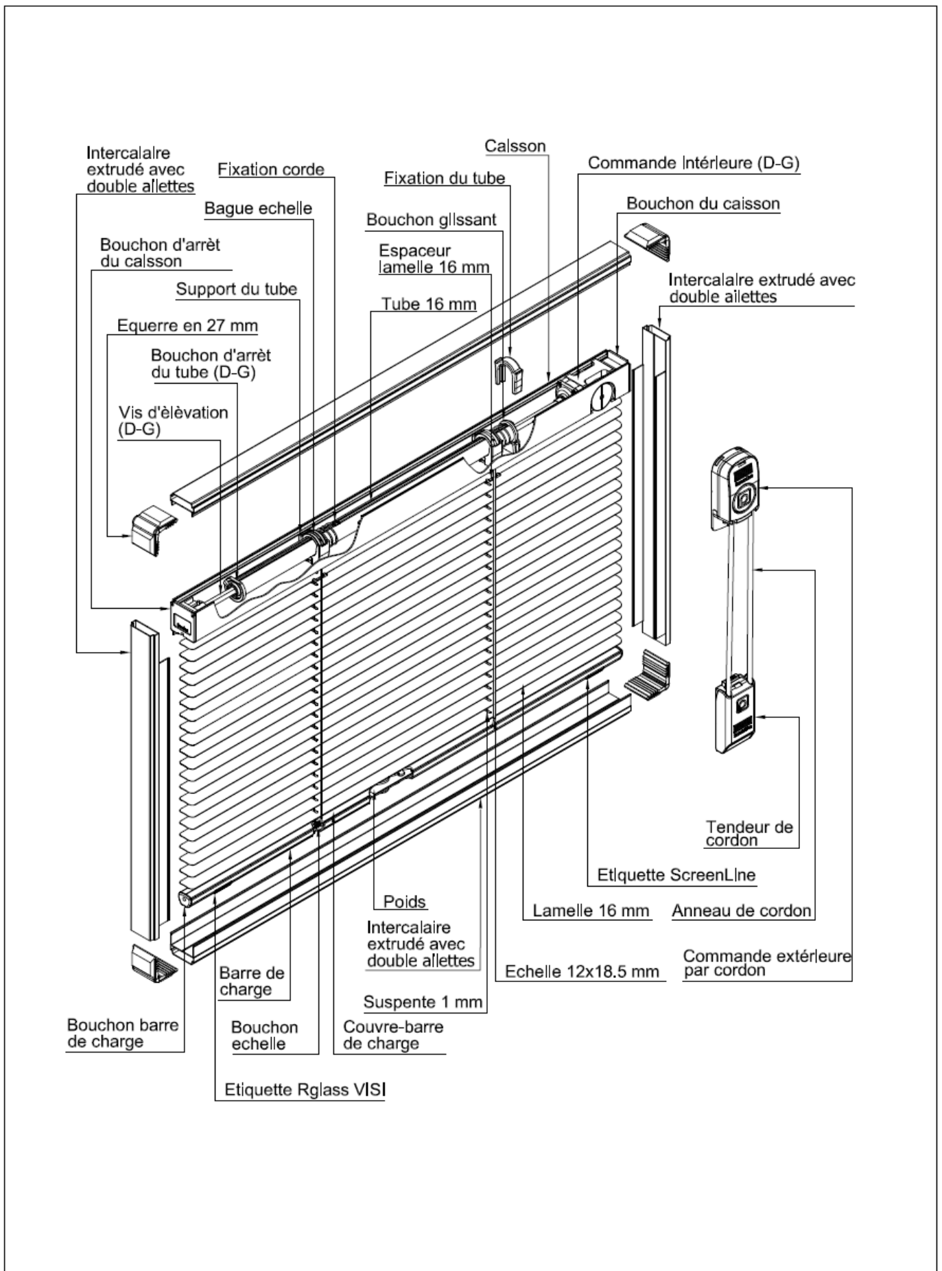
Figure 1 - Vue d'ensemble éclatée
