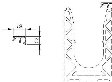
Figure 10 – Petit capot pour modèle SABCO 007011, SABCO 007012, SABCO 007013
