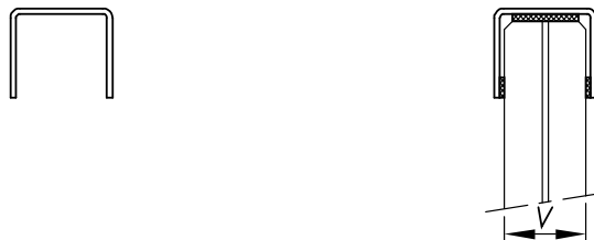
Figure 23 – Main courante pour tous les modèles SABCO (V correspond à l'épaisseur du vitrage utilisé).
