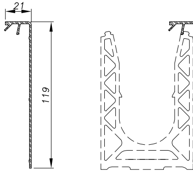
Figure 9 – Grand capot pour modèle SABCO 007010, SABCO 007011
