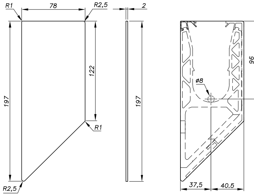
Figure 20 – Réf : 007013PLA – Bouchon (à percer Ø 8 pour le drainage si nécessaire)
