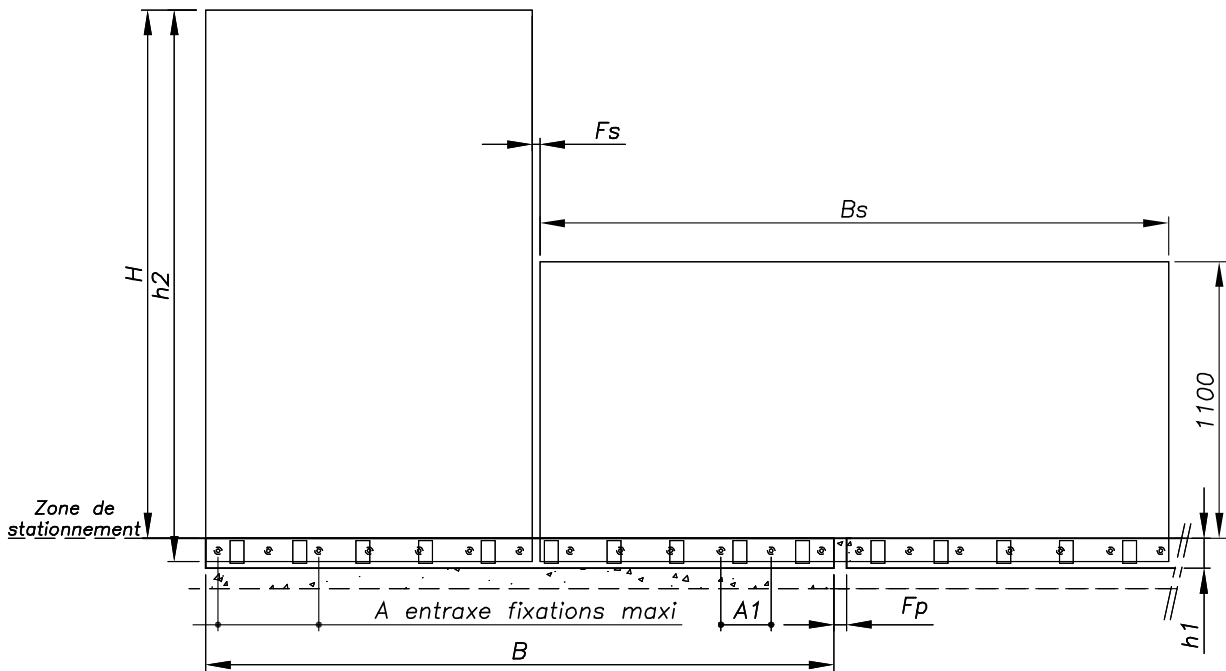
Figure 4 - Montage en nez de dalle - Modèle SABCO 007011
