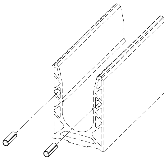
Figure 15 – Goupille de jonction
