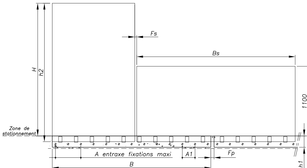
Figure 6 - Montage en nez de dalle - Modèle SABCO 007013
