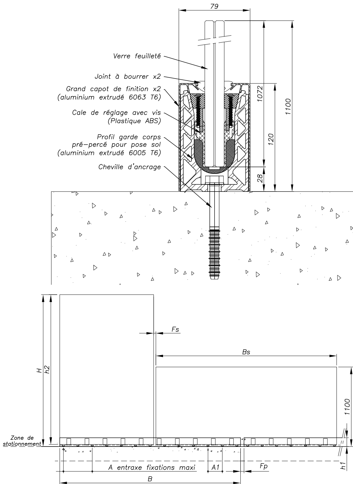
Figure 3 - Montage au sol - Modèle SABCO 007010
