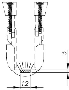
Figure 24 – Encombrement pour LED
