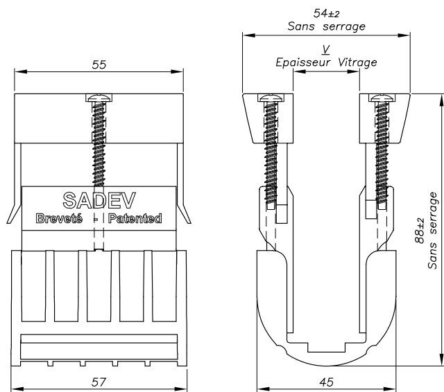
Figure 13 – Cale pour modèle SABCO 007010, SABCO 007011, SABCO 007012, SABCO 007013
