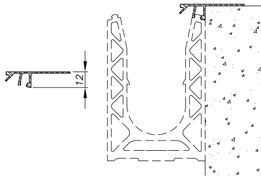
Figure 10 – Petit capot pour modèle SABCO 007011, SABCO 007012, SABCO 007013
