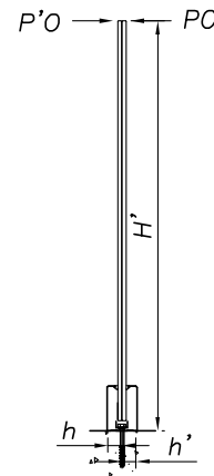
Figure 1 – Dimensionnement des chevilles fixation au sol
