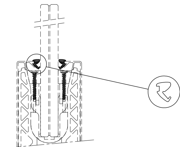
Figure 14 – Joint pour modèle SABCO 007010, SABCO 007011, SABCO 007012, SABCO 007013
