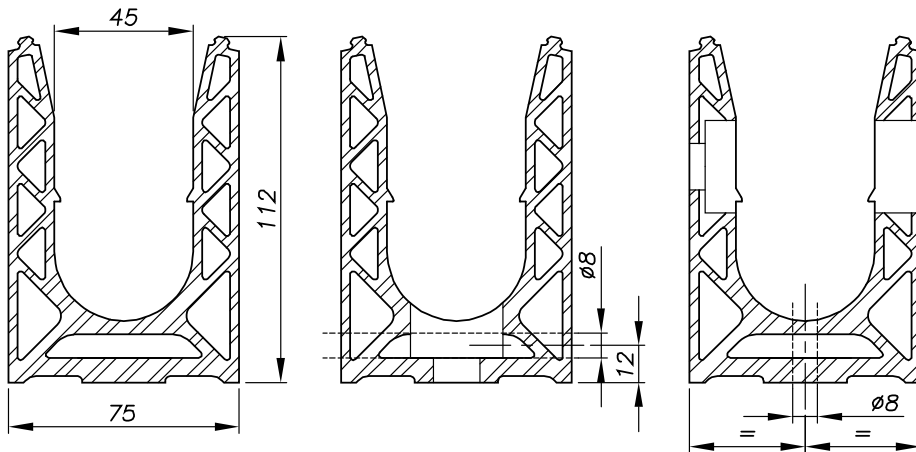
Figure 7 - Profil pour modèle SABCO 007010, SABCO 007011, SABCO 007012 (à percer Ø 8 pour le drainage si nécessaire)
