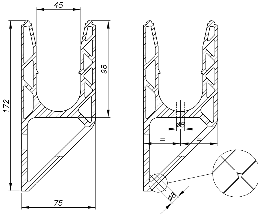
Figure 8 - Profil pour modèle SABCO 007013 (à percer Ø 8 pour le drainage si nécessaire)
