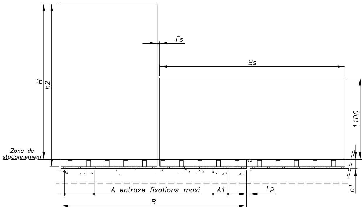
Figure 5 - Montage au sol - Modèle SABCO 007012
