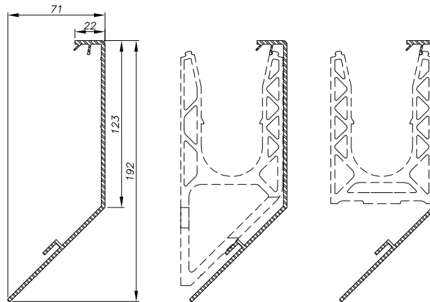
Figure 12 – Grand capot pour modèle SABCO 007013, SABCO 007011
