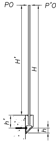
Figure 2 – Dimensionnement des chevilles fixation nez de dalle
