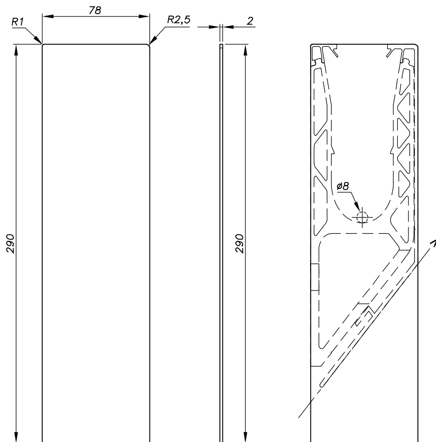
Figure 21 – Réf : 007013PLARAM - Bouchon à recouper en hauteur (à percer Ø 8 pour le drainage si nécessaire)
